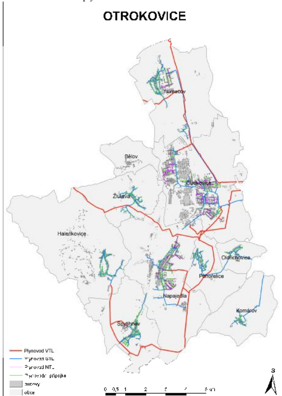
Obrázek: Zásobování plynem SO ORP Otrokovice
