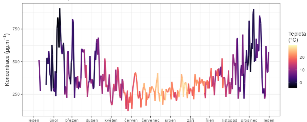
Vývoj maximálních 8h koncentrací CO za den v závislosti na teplotě vzduchu Otrokovice - město, rok 2023
