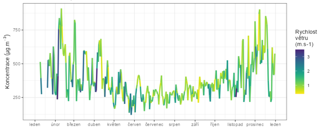
Vývoj maximálních 8h koncentrací CO za den v závislosti na rychlosti větru Otrokovice - město, rok 2023
