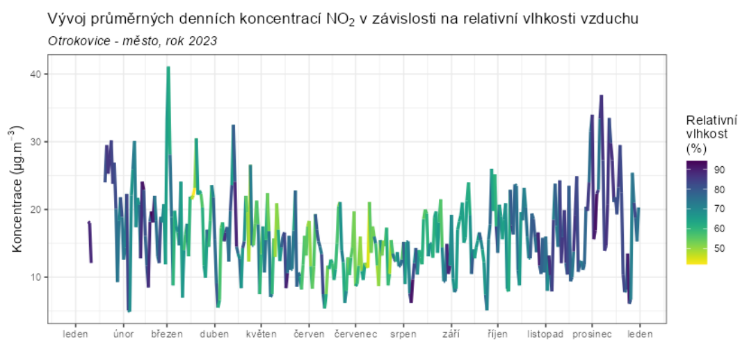
Obr. 42 – Vliv teploty (nahore), rychlosti větru (uprostřed) a relativní vlhkosti (dole) na koncentrace NO 2 , Otrokovice – město, rok 2023
