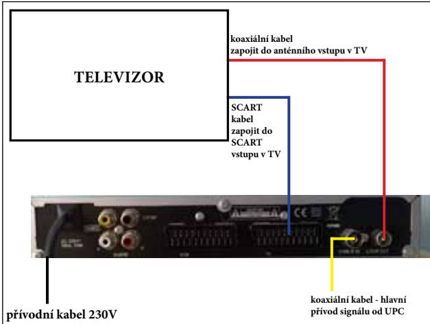
Schéma zapojení příslušných kabelů do set-top-boxu a televizoru v případě připojení u společnosti UPC.
